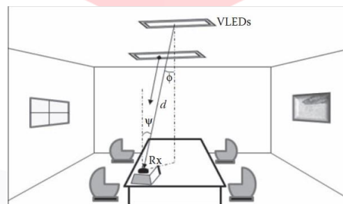
Gambar 2.1. Ilustrasi FWHM
