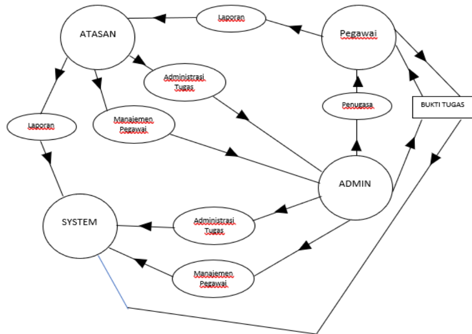
Gambar 4 Diagram aktor.
