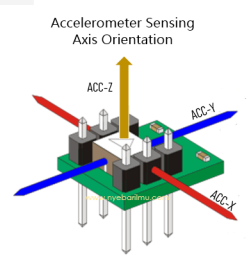
Gambar 2.3. Ilustrasi Accelerometer.
