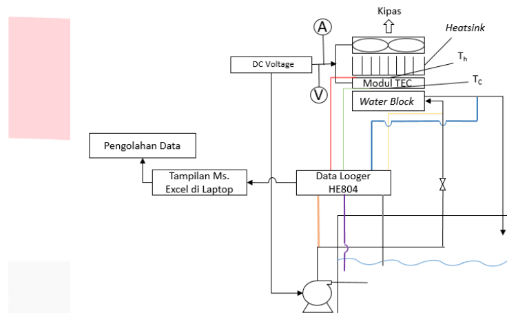
Gambar 2.3 Skema pengukuran penelitian
