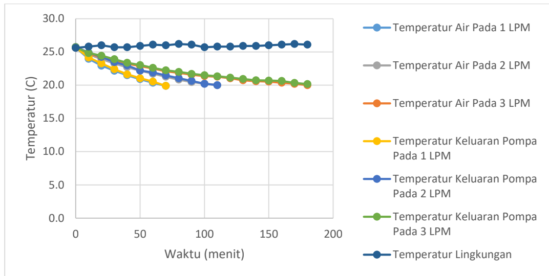
Gambar 3.1 Grafik Perubahan Temperatur Pada Berbagai Variasi Laju Aliran
