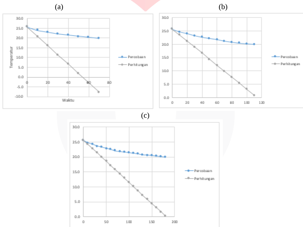
Gambar 3.4 Penurunan Temperatur Pada (a) 1LPM, (b) 2LPM, dan (c) 3 LPM
