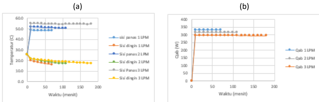
Gambar 3.3 (a) Temperatur sisi panas dan dingin TEC (b) nilai penyerapan kalor oleh sisi dingin TEC ( \dot{Q}_{ab} )
