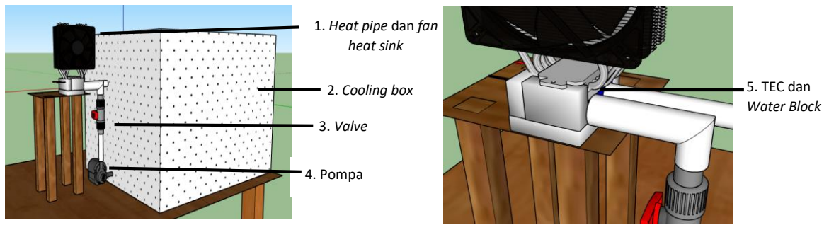
Gambar 2.2 Perancangan sistem pendingin
