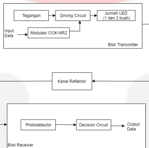
Gambar 2. 1 Blok Desain Sistem untuk VLC.
