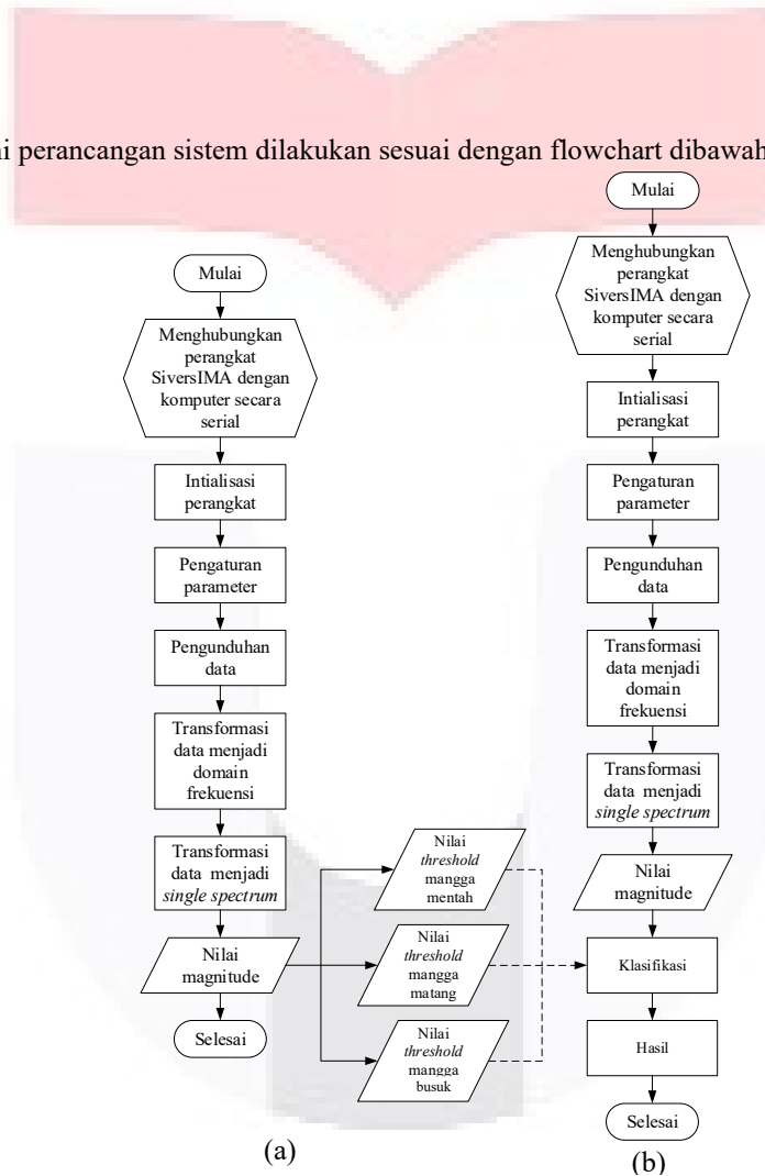
Gambar 3. Flowchart sistem deteksi kematangan mangga. (a) proses pencarian level threshold . (b) proses klasifikasi tingkat kematangan.
