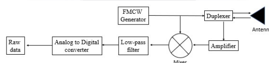
Gambar 1. Sistem dasar pada FMCW.
