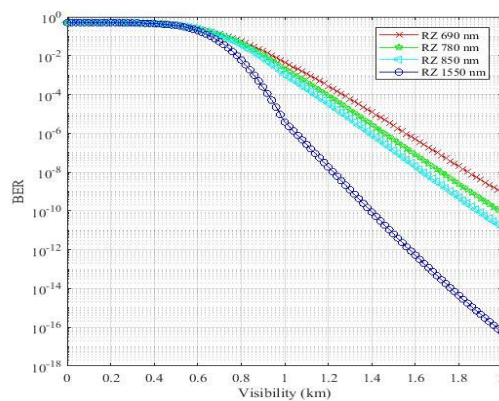
Gambar 5 Grafik BER OOK-RZ pada Kanal Kim
