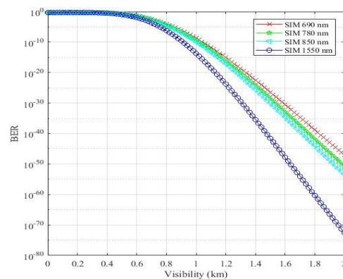
Gambar 6 Grafik BER SIM pada Kanal Kruse
