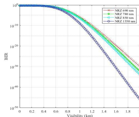
Gambar 7 Grafik BER OOK-NRZ pada Kanal Kruse
