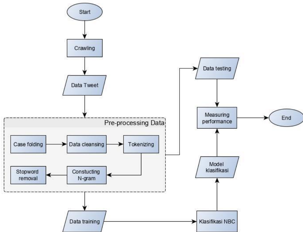
Gambar 1 Flowchart Klasifikasi Sentimen
