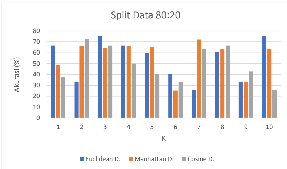
Gambar 7. Grafik hasil split data 80:20
