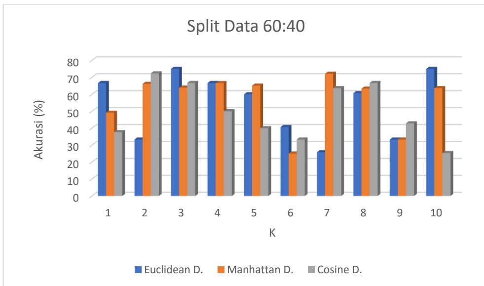
Gambar 5. Grafik hasil split data 60:40
