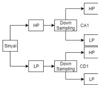
Gambar 4. Dekomposisi Sinyal
