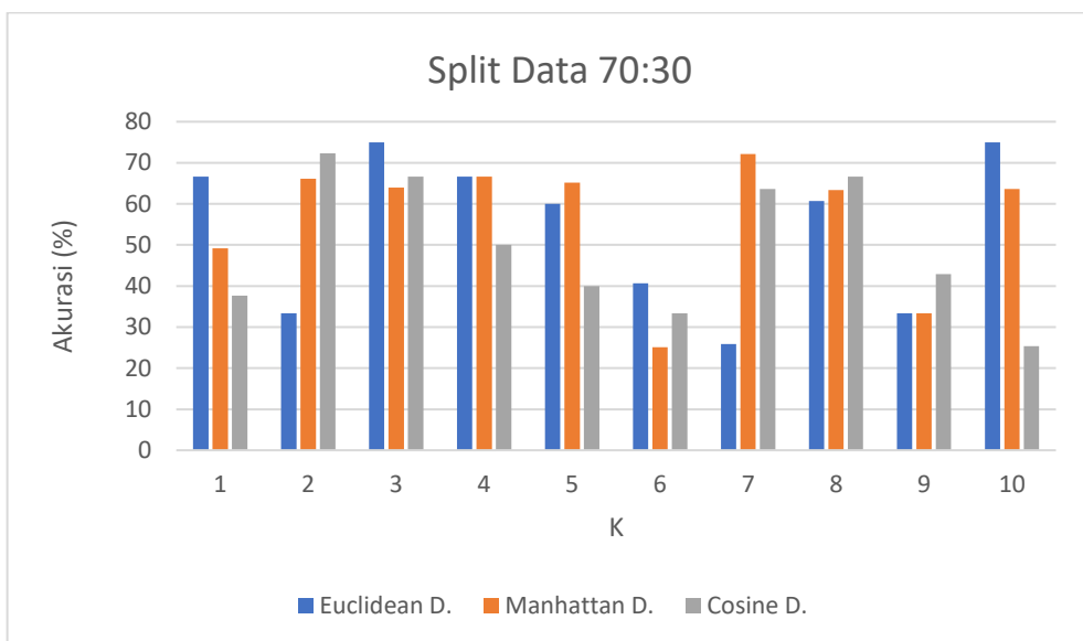
Gambar 6. Grafik hasil split data 70:30
