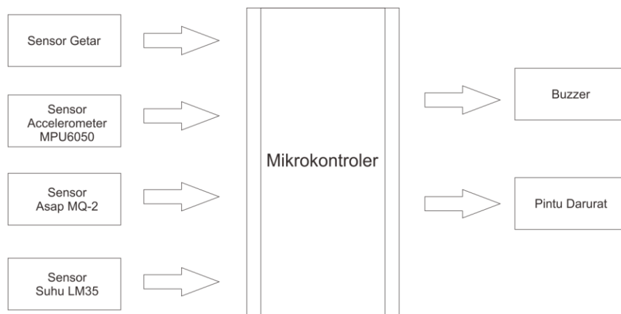
Gambar 3 Diagram Blok Perancangan Sistem
