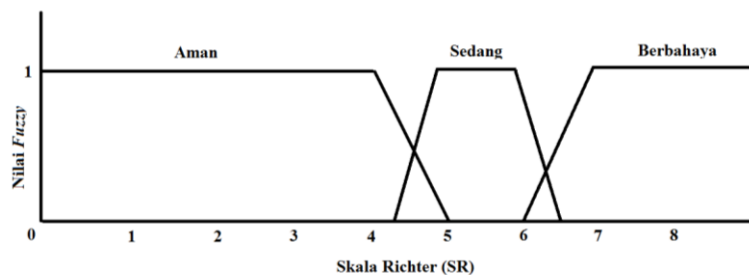
Gambar 6 Fungsi Keanggotaan Gempa
