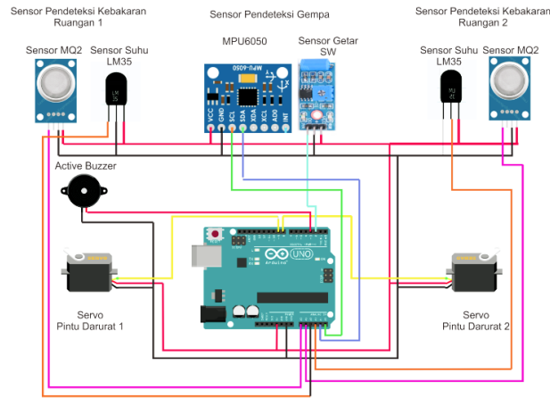
Gambar 4 Rangkaian Sistem
