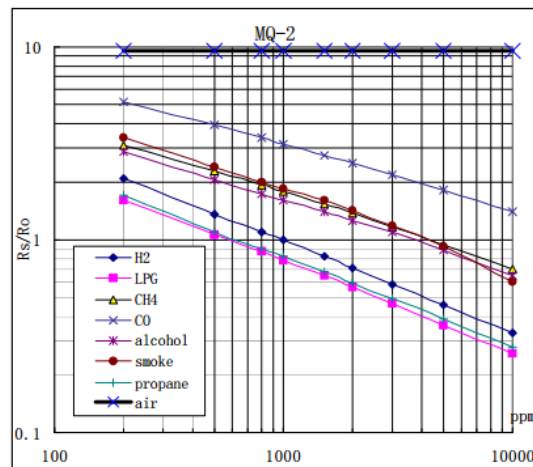
Gambar 1 Karakteristik Sensitivitas MQ-2
