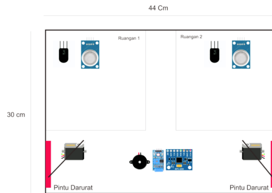
Gambar 5 Desain Prototipe
