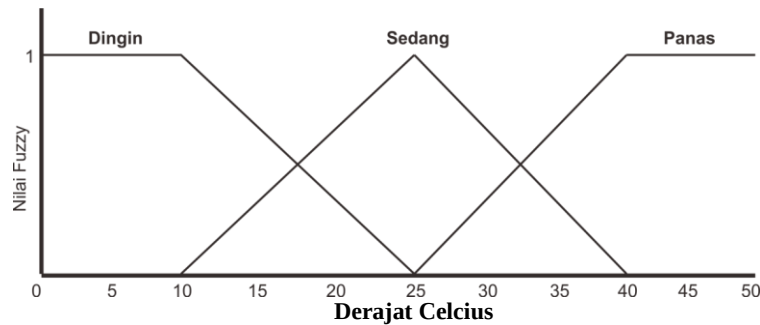
Gambar 7 Fungsi Keanggotaan Suhu
