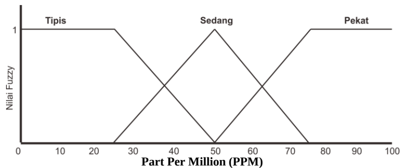
Gambar 8 Fungsi Keanggotaan Asap
