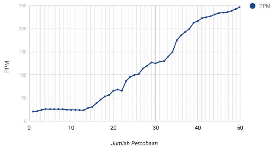
Gambar 12 Pembacaan Sensor MQ2 (Kondisi penuh asap)
