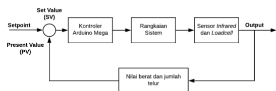
Gambar 3. 3 Diagram Blok sistem
