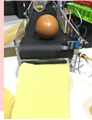
Gambar 4. 6 Prototipe Penghitung Jumlah Telur
