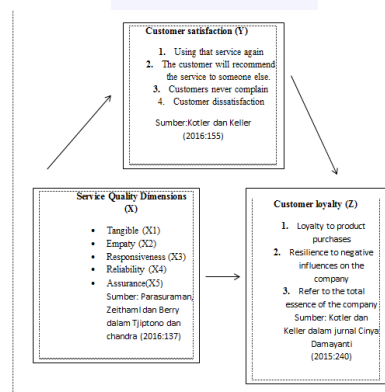
Gambar 1 Kerangka Pemikiran
