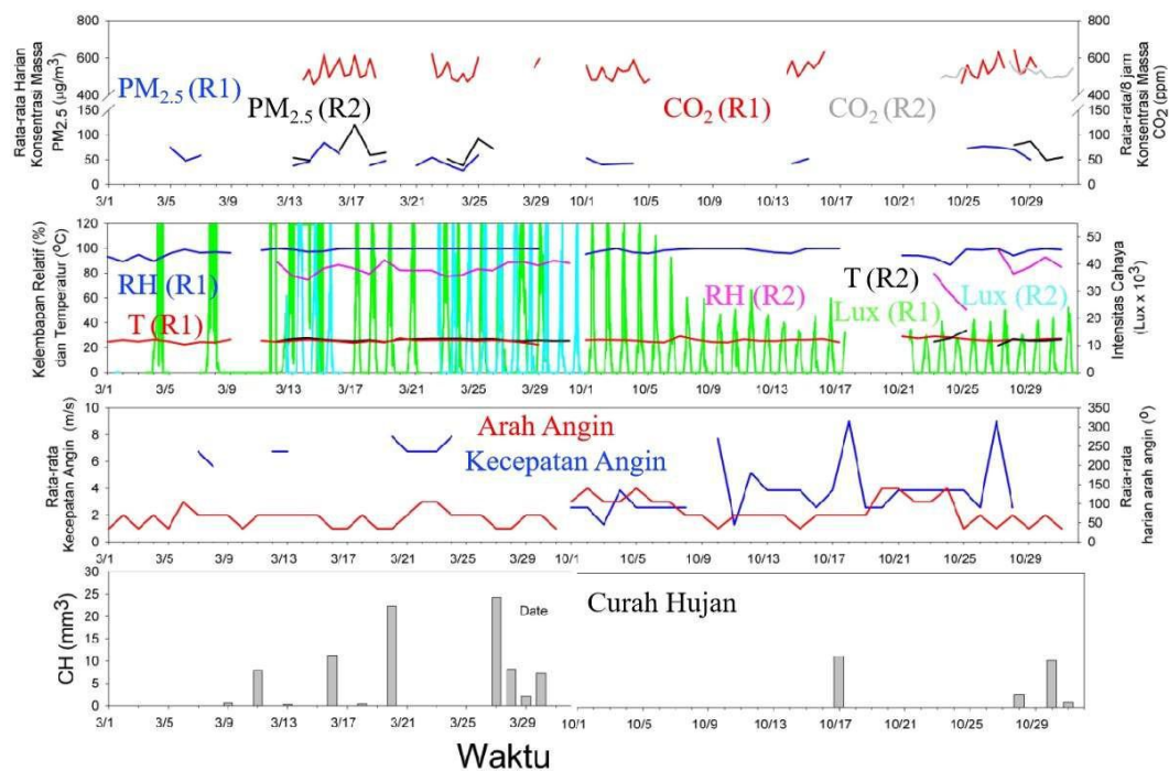
Gambar 5. Rata-rata konsentrasi polutan PM_{2.5} , CO_2 , dan parameter meteorologi ( T , RH , I , WS , WD , curah hujan) di musim pancaroba.
