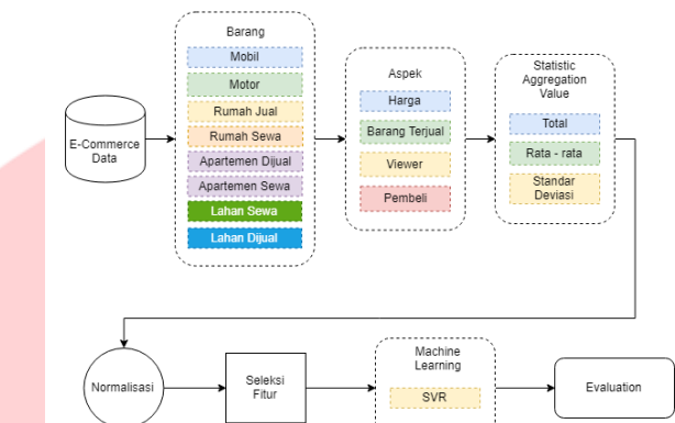
Gambar 6 Gambar Alur Pengolahan Data Menggunakan Machine Learning
