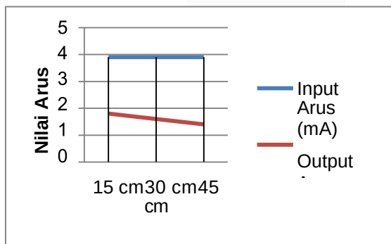
Gambar 4.3 Grafik Respon Penerima sudut 10^{\circ}
