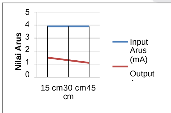
Gambar 4.3 Grafik Respon Penerima sudut 10^{\circ}
