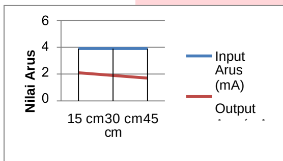
Gambar 4.2 Grafik Respon Penerima sudut 0^{\circ}
