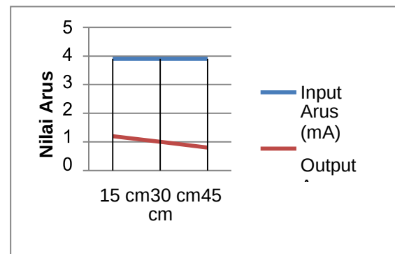
Gambar 4.5 Grafik Respon Penerima sudut 30^{\circ}
