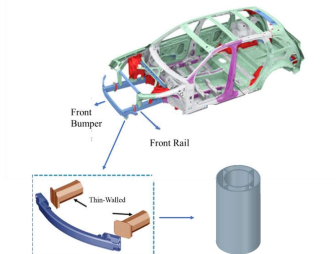
Gambar 1 Penerapan struktur Thin-Walled pada sasis kendaraan roda empat
