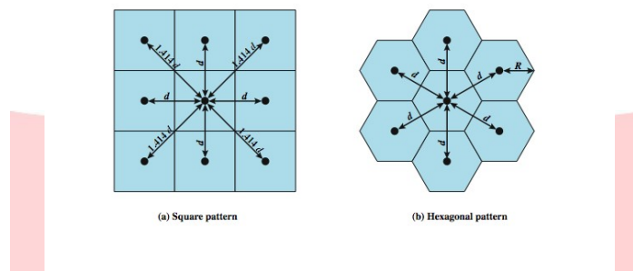
Gambar 2. 1 Pembagian Area pada jaringan seluler
