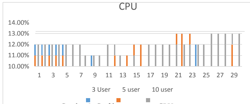
Gambar 2. Grafik penggunaan CPU server.
