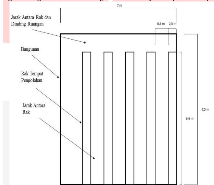
Gambar 1. 2 Layout Ruang Pengolahan Kotoran Ayam
