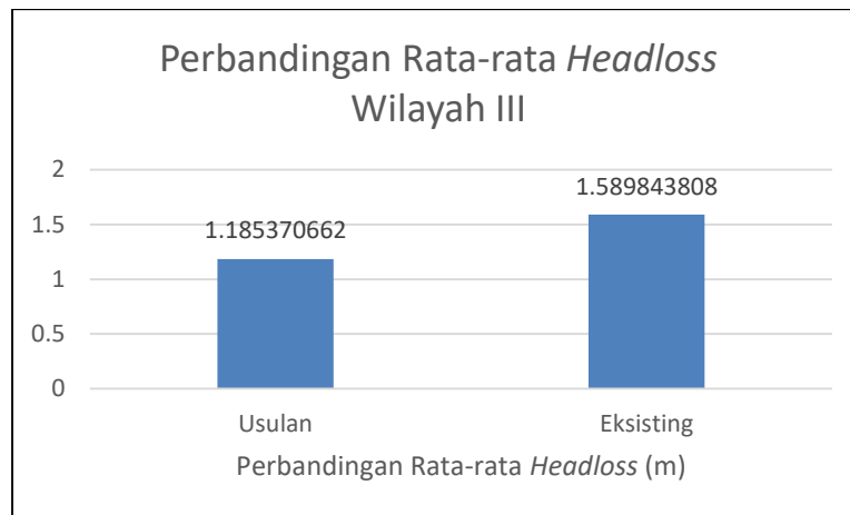
Gambar 12 Perbandingan Rata-rata Headloss Wilayah 3
