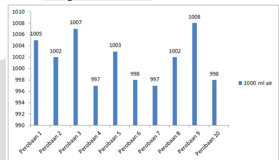
Gambar 4. 7 Pengujian debit air
