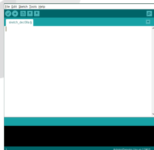
Gambar 2. 7 Arduino IDE
