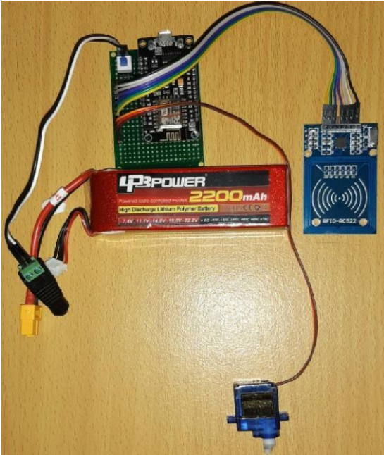
Gambar 4.2 Skema PA Pengujian
