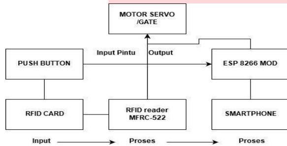
Gambar 3.3 Blok diagram perancangan sistem
