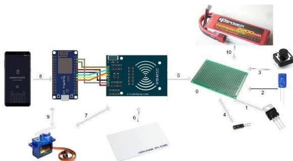
Gambar 4.1 Skema PA
