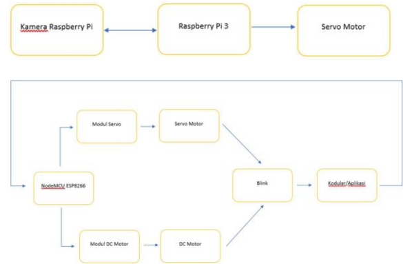
Gambar 3.1 Blok Diagram Raspberry Pi 3 dan NodeMCU ESP8266
