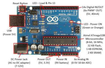
Gambar 2. 3 Arduino Uno.
