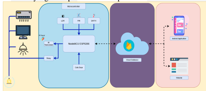
Gambar 1 Desain Sistem
