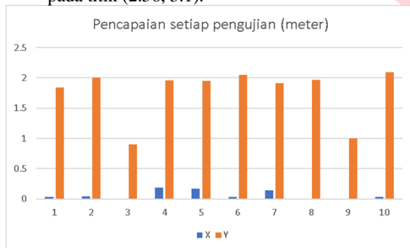
Gambar 4.11. Grafik Pencapaian Titik Akhir Kursi Roda Dari Setiap Percobaan, titik awal (2.3, -1.3) meter.
