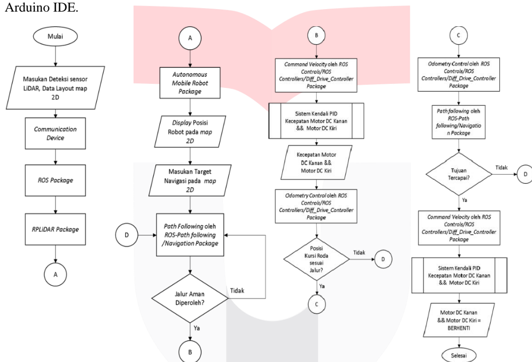
Gambar 3.3. Diagram Alir
