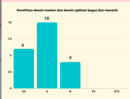
Gambar 4.1 Grafik Pertanyaan 1
