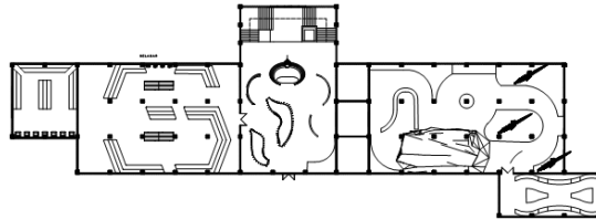
Gambar 6 Layout khusus lantai 1 sumber: dokumentasi penulis
