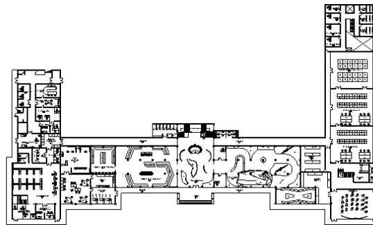
Gambar 4 Layout general lantai 1 sumber: dokumentasi penulis
