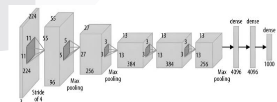
Gambar 2. 3 Arsitektur Alexne
