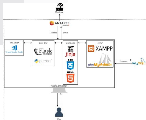
GAMBAR 1 ARSITEKTUR APLIKASI.
