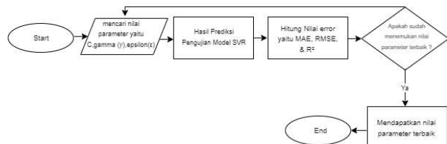
GAMBAR 3.5 DIAGRAM ALIR MENDAPATKAN ANGKA PARAMETER TERBAIK DENGAN ALGORITMA GRID SEARCH
