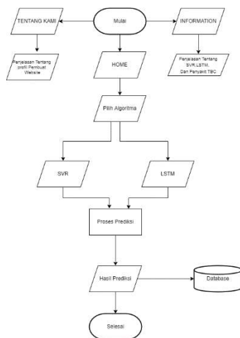
GAMBAR 3.1 GAMBARAN UMUM SISTEM
