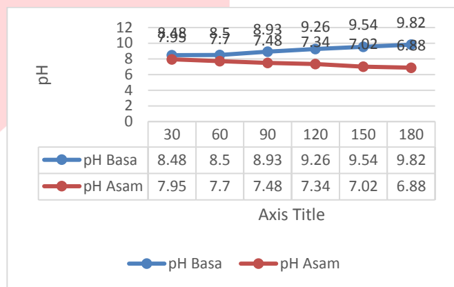
Gambar 12. Grafik Pengujian Sistem Water Ionizer kedua
