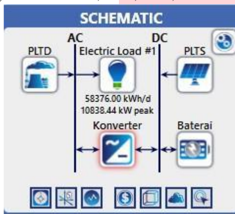
Gambar 3 Skematik Eksisting
