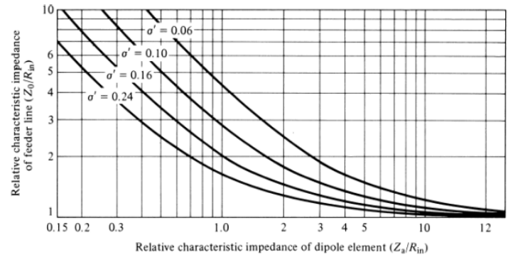
GAMBAR 2 KONTUR DIREKTIVITAS KONSTAN PERBANDINGAN \Sigma DAN UNTUK LDPA[7]
