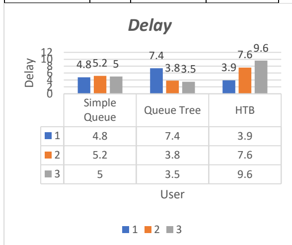
Gambar 15. Grafik Delay
