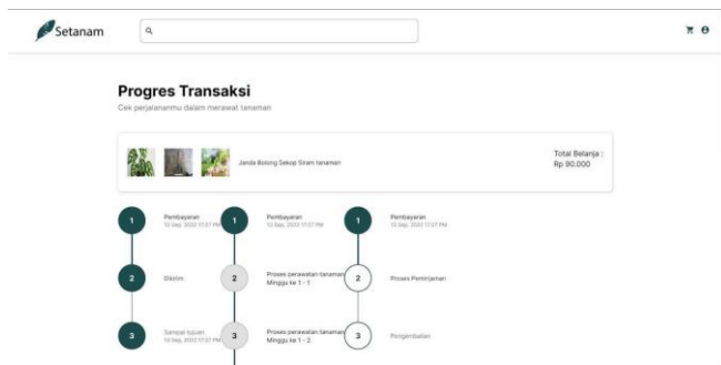
GAMBAR 15 PROGRES TRANSAKSI
