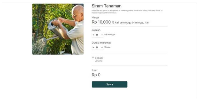
GAMBAR 13 DETAIL PRODUK
