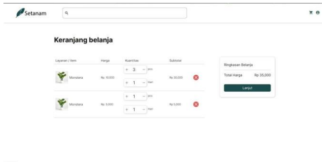
GAMBAR 14 KERANJANG BELANJA
