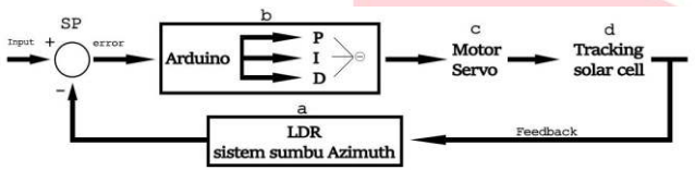
Gambar 3 – 4 Metode PID
