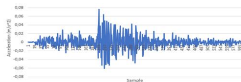
GAMBAR 9 Sinyal Yang Terbentuk Pada Truk Melintas
