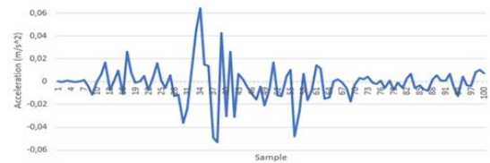
GAMBAR 5 Sinyal Gempa Sebelum Downsampling
