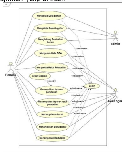
GAMBAR 3- 2 Ilustrasi Usecase Diagram.
