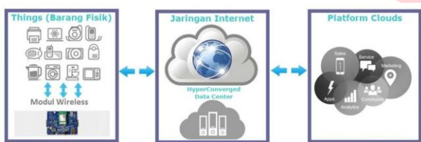
GAMBAR 2.2 Arsitektur IoT
