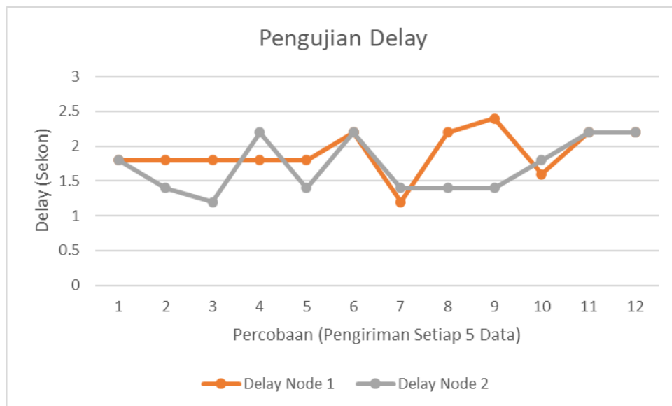
Gambar 4. 8 Grafik Penguujian Delay Sensor Node 1 dan Sensor Node 2
