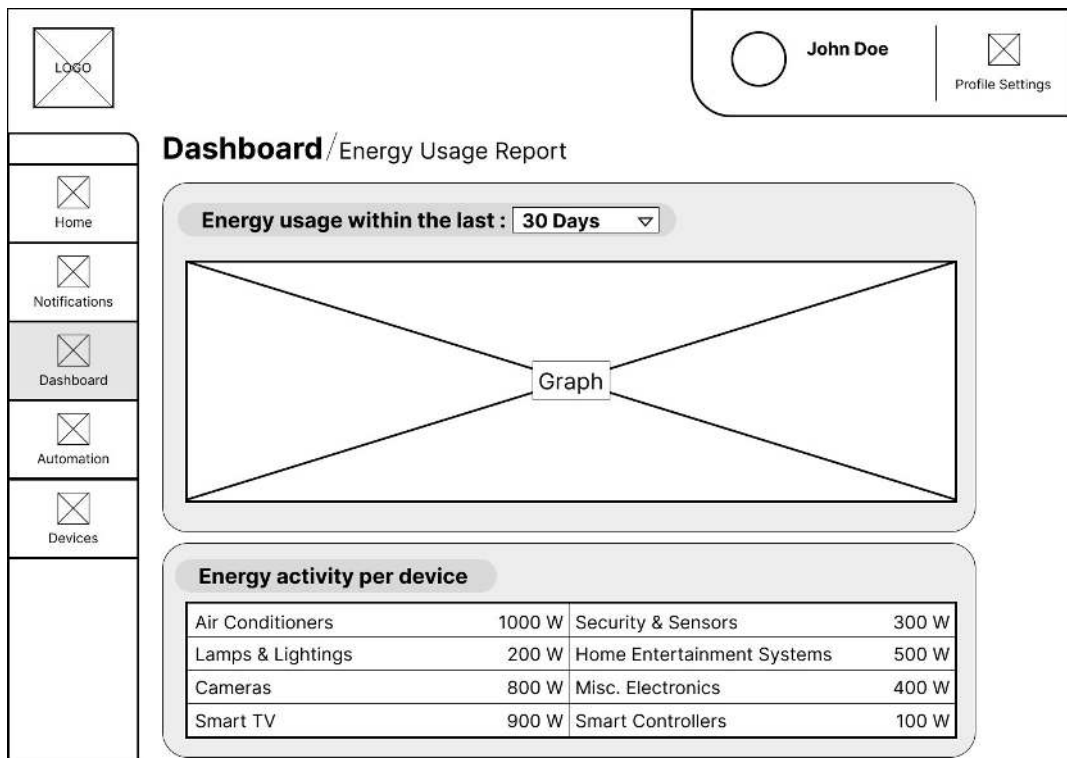
Gambar 19 Wireframe Dashboard
