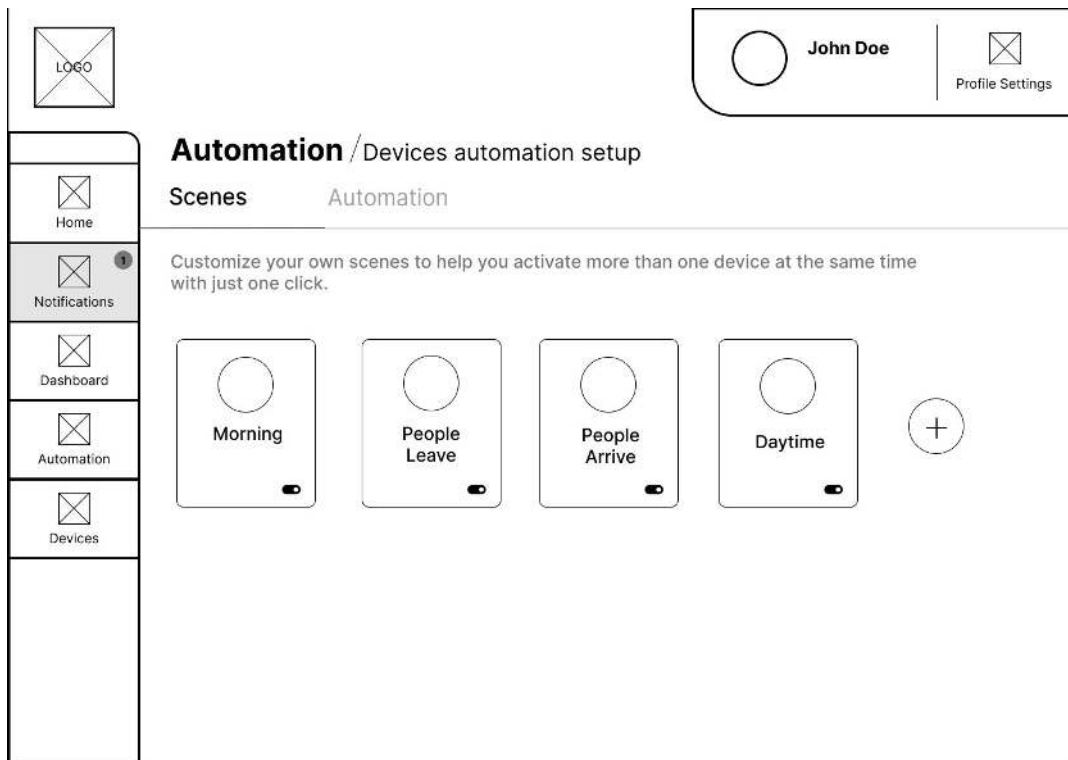
Gambar 25 Wireframe Automation 1
