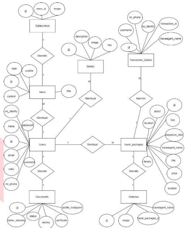
GAMBAR 3.2 Artistektur Aplikasi
