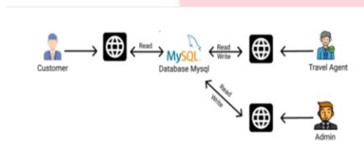
GAMBAR 3.1 Arsitektur aplikasi
