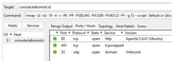
GAMBAR 4.1 Hasil Pengujian Nmap
