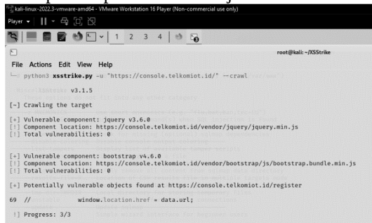
GAMBAR 4.5 Hasil Pengujian XSS menggunakan XSSStrike
