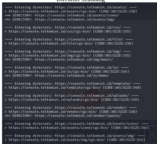
GAMBAR 4.3 Direktori Scanning
