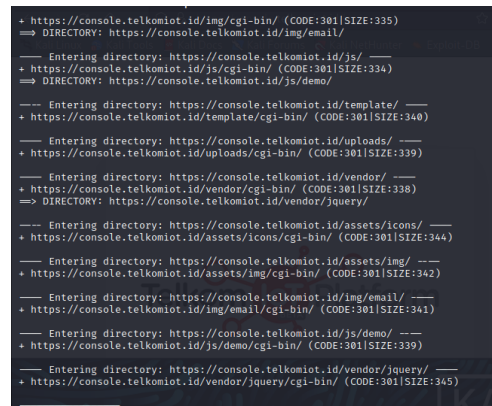
GAMBAR 4.4 Direktori Scanning
