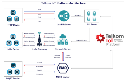
GAMBAR 3.1 Arsitektur Telkom IoT Platform
