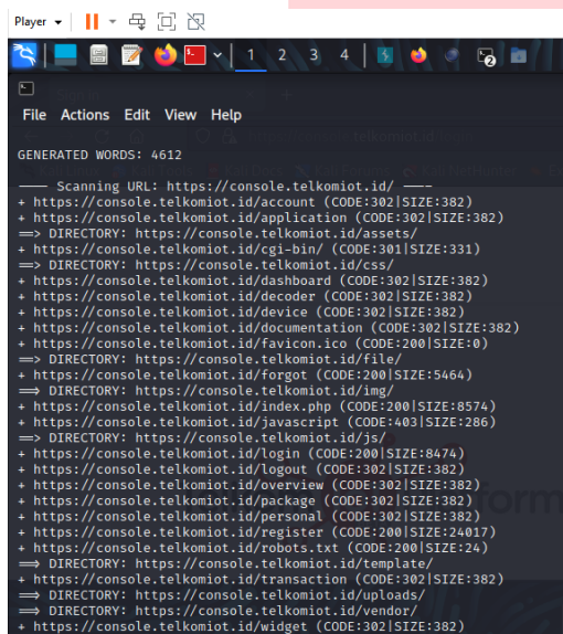
GAMBAR 4.2 Direktori Scanning
