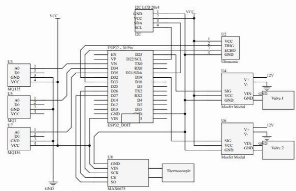
Gambar 3.1 Wiring Sensor ke ESP32
