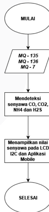
GAMBAR 3.2 Flowchart pembacaan senyawa
