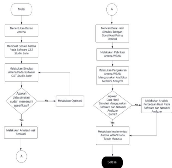
GAMBAR 1. Flowchart Pembuatan Antena WBAN
