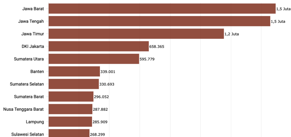
Gambar 1. 5 Jumlah UMKM
