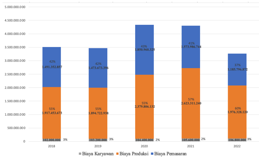
Gambar 1. 8 Grafik Biaya
