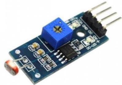
GAMBAR 2 (Sensor LDR)
