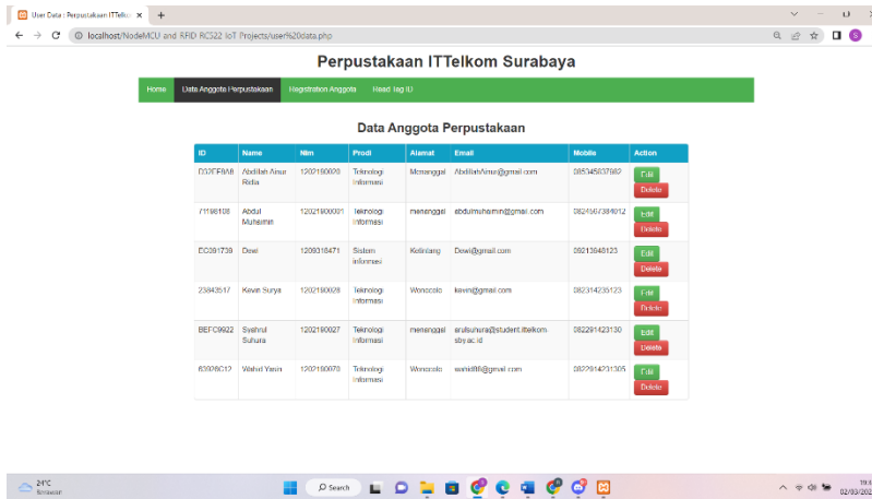
Gambar 14. Data Anggota
