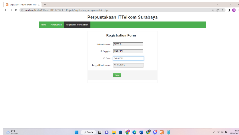
Gambar 15. Registrasi Peminjaman
