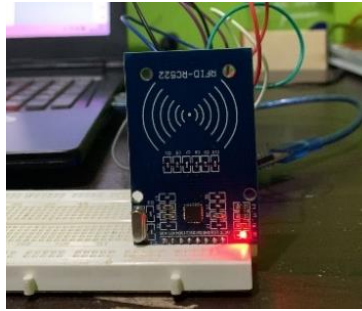
Gambar 10. Alat RFID
