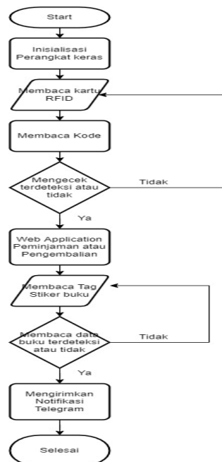
Gambar 3. Diagram Alir Sistem
