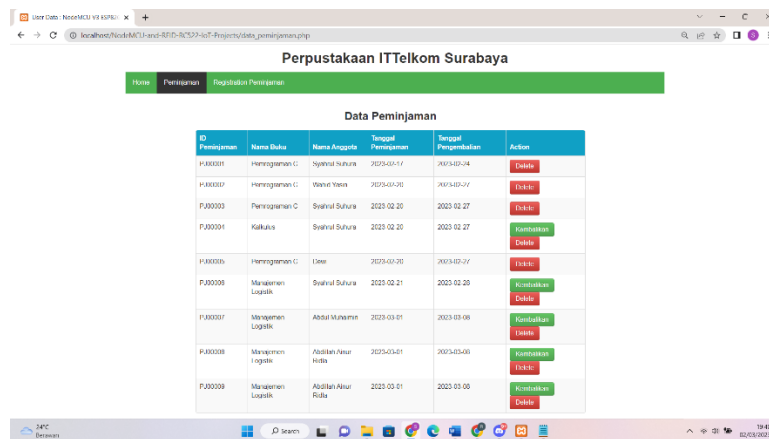
Gambar 16. Data Peminjaman
