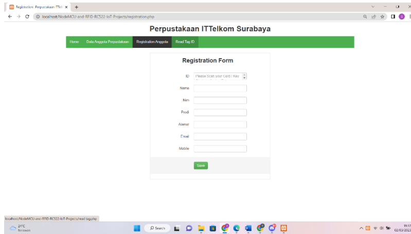
Gambar 13. Registrasi Anggota
