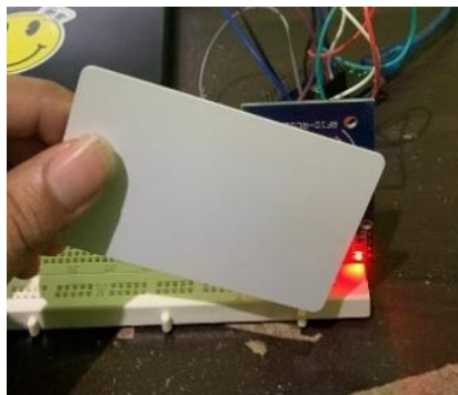
Gambar 11. Scan Kartu
