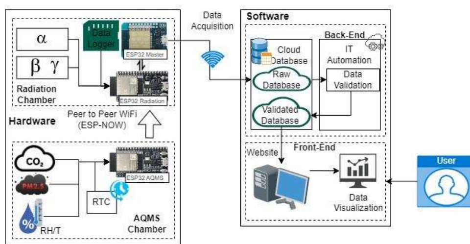
Gambar 1.4. Blok Diagram Sistem
